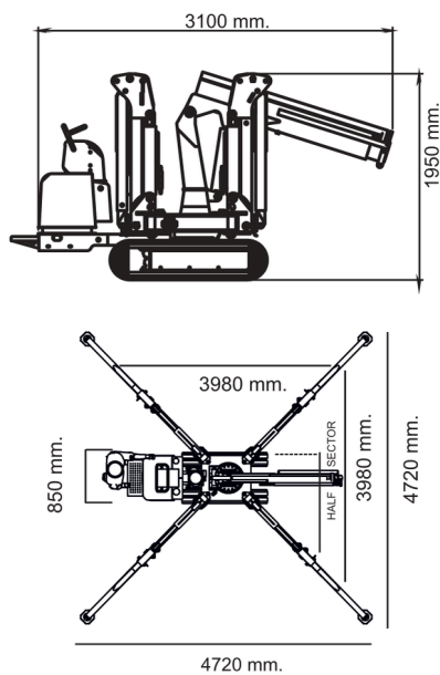
Dimensioni Generali - Generals Dimensions - Dimensions Générales Gesamtmaßungen - Dimensiones Generales
